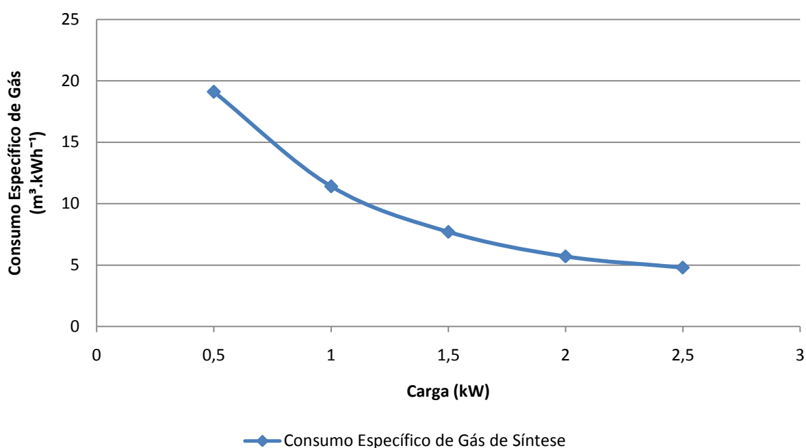
Figura 17- Consumo específico de gás de síntese.
