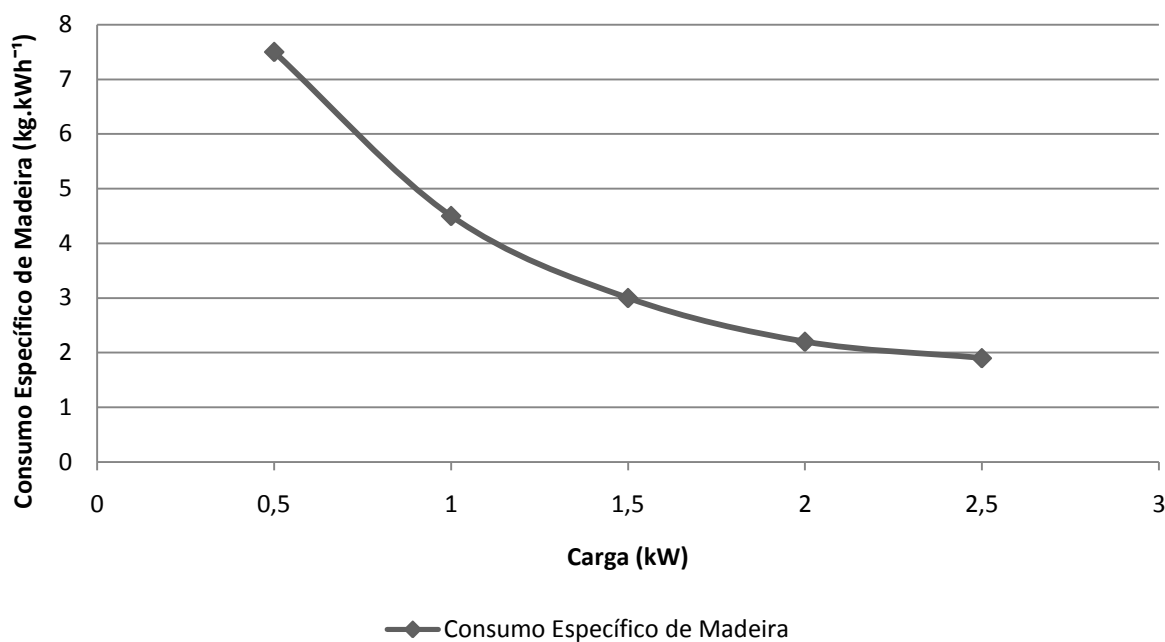
Figura 18 - Consumo específico de madeira.
