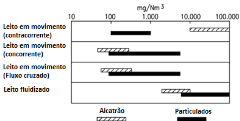
Figura 5- Concentração de alcatrão e particulados produzido em gaseificadores (GUIGON & LARGE, 1990).
